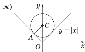
Два решения AC = OA = 1, OC = a = \sqrt{2}
